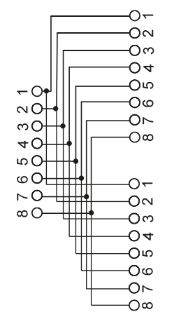
Beschaltung pinout
