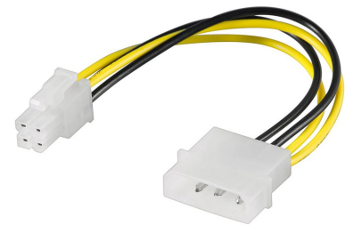
Cable alimentación 4 pins a IDE
