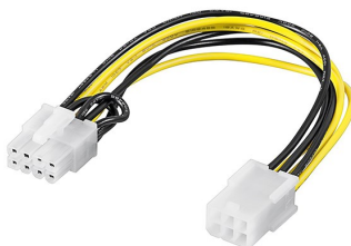
Adaptador alimentación PCI 6P A 8
