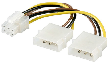
Adaptador alimentación PCI a 2 x IDE
